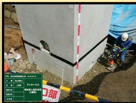
排水構造物埋戻し状況
