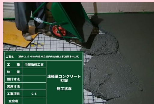
A棟4階 男子トイレ 土間コンクリート打設状況
