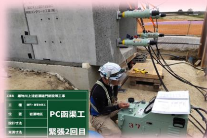
PC函渠 緊張状況
