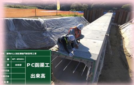
函渠工（PC函渠）完了
