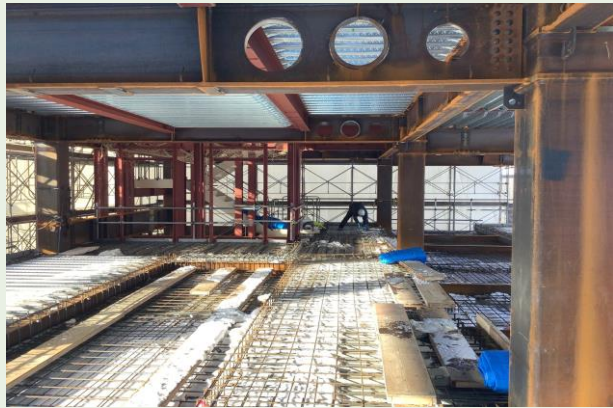
6階 スラブ配筋状況
