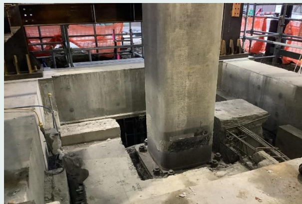
ジャッキ架台基礎 型枠解体状況
