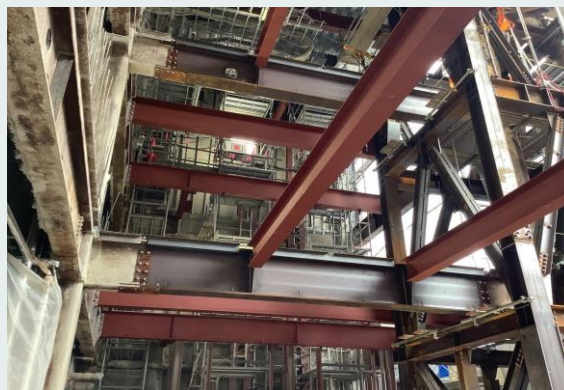
鉄骨柱復旧状況
