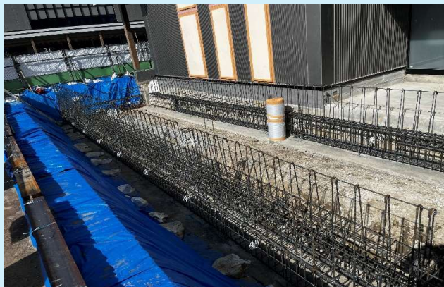
B-1棟 基礎配筋状況
