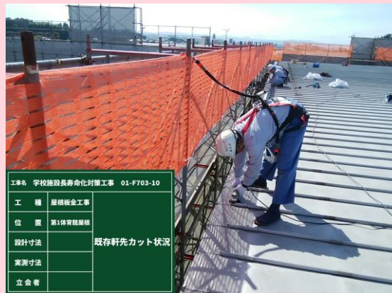
第一体育館 既存軒先カット
